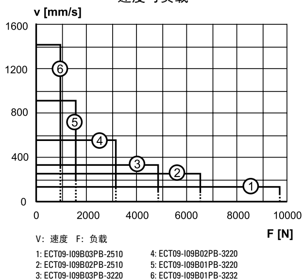
速度与负载
