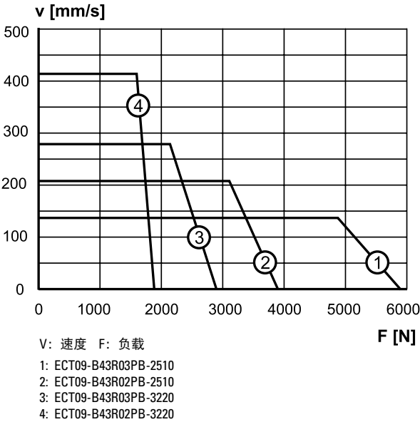
速度与负载
