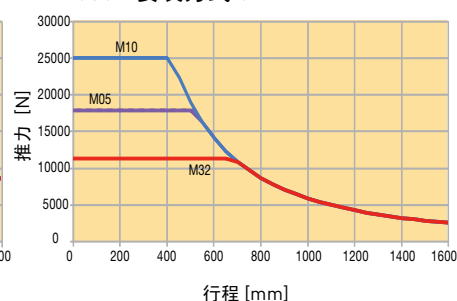
ETH080 - 安装方式 3
