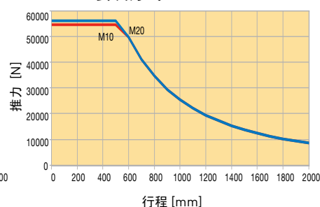
ETH100 - 安装方式 3
