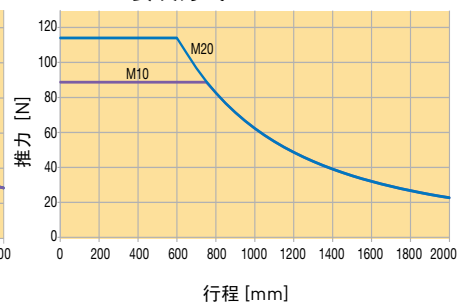
ETH125 - 安装方式 3
