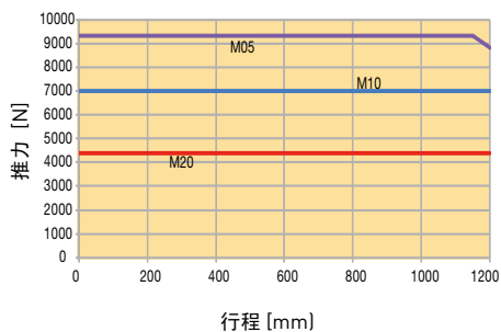
ETH050 - 安装方式 1
