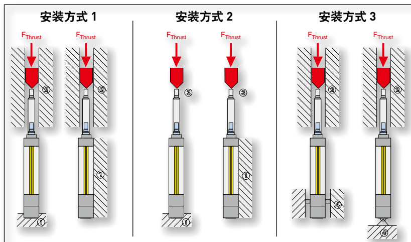
ETH080 - 安装方式 2
