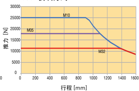
ETH080 - 安装方式 2
