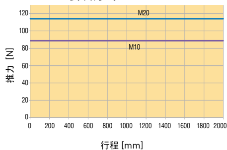
ETH125 - 安装方式 1
