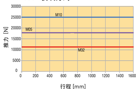
ETH080 - 安装方式 1
