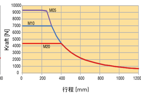
ETH050 - 安装方式 3
