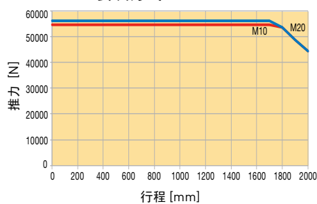
ETH100 - 安装方式 1
